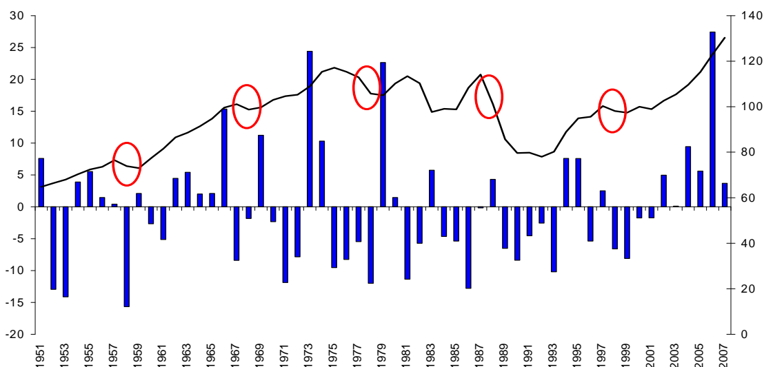
Gráfico 1 PBI PERCÁPITA Y TÉRMINOS DE INTERCAMBIO: 1951 - 2007
