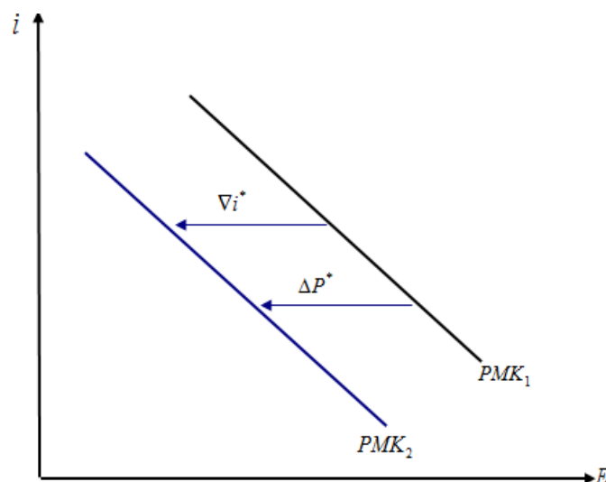
Figura 2: La Curva PMK
