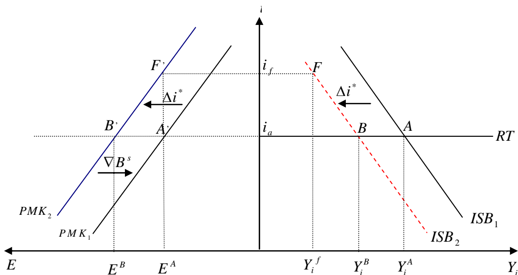
Figura 7: como enfrentar una salida de capitales ( i^* sube)
