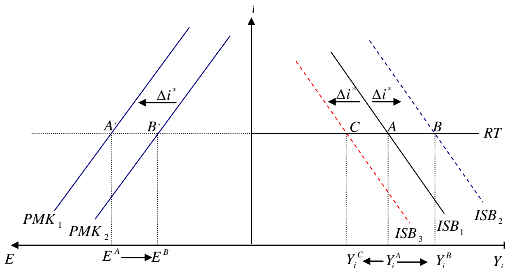
Figura 6: i^* cae con tipo de cambio flotante
