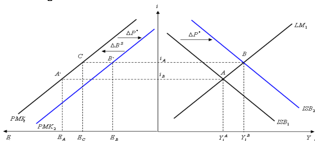
Figura 5: P^* sube con intervención esterilizada
