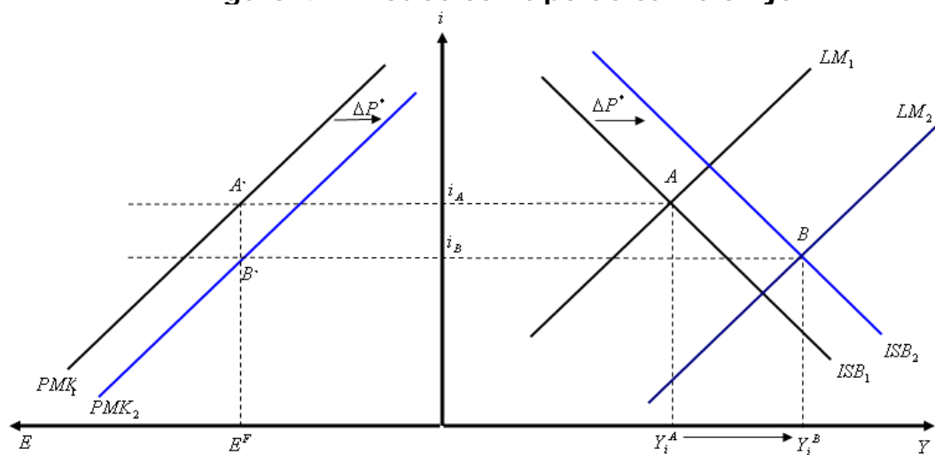
Figura 4: P^* sube con tipo de cambio fijo
