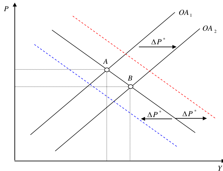
Figura 8: alza del precio de las materias primas ( P^* ) traslada las curvas de demanda agregada y de oferta agregada.
