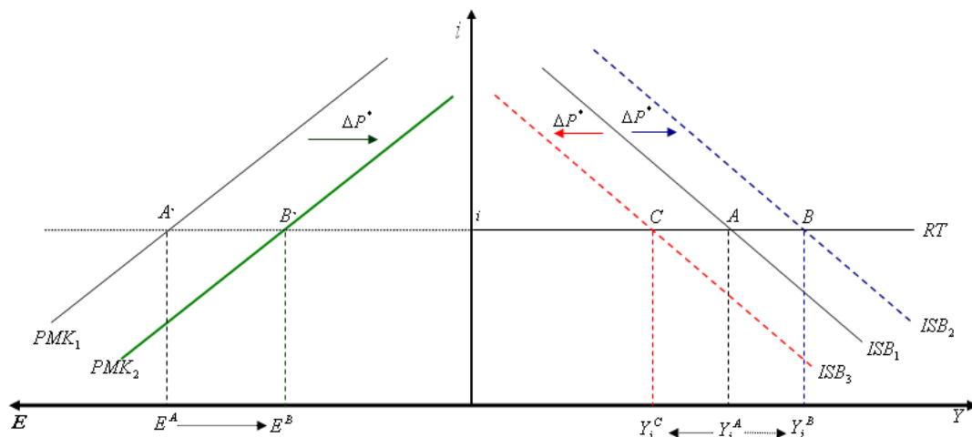
Figura 3: P^* sube con tipo de cambio flotante
